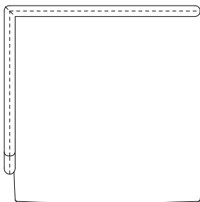
poltrona C238 1BR ESQUERDO 90x90x65cm (LxPxA) almofadas: 1x und. decorativa 50x50cm 1x und. decorativa 55x55cm
