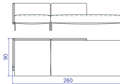
poltrona C238 1BR esquerdo | 95 x 90 x 65cm (LxPxA) sofá C138 SBR ER direito | 170 x 90 x 65cm (LxPxA)
