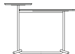
mesa lateral: 80x30x55cm (LxPxA)
